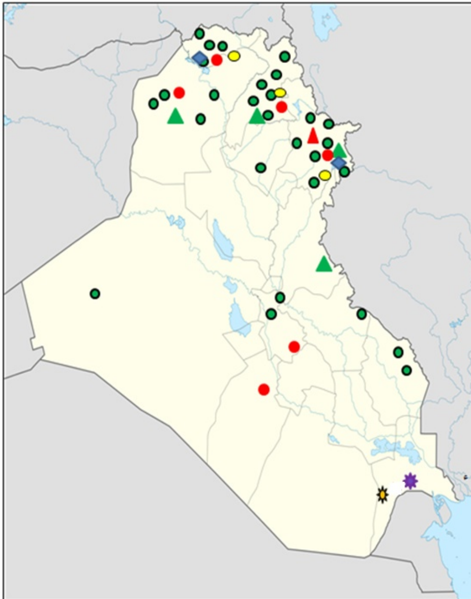
Fig. 1: Distribution in Iraq of ● P. aegyptiaca , ● P. coelistes , ✪ P. hypertomentosa , ● P. mutelii , ✪ P. nama , ▲ P. ramosa , ◆ P. orientalis , ▲ P. oxyloba , ✪ P. umqasrensis
